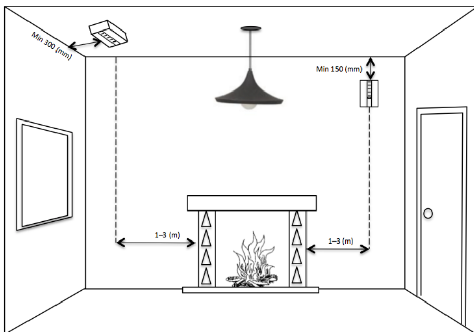
Afbeelding 1: ruimte met verbrandingsapparaat
